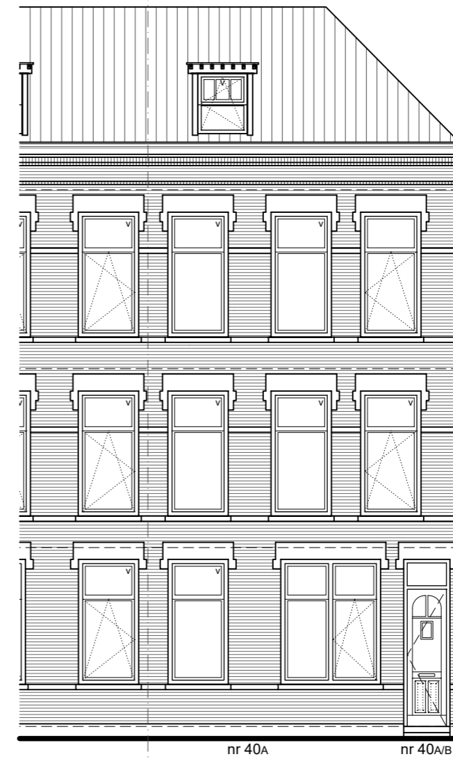
rechter zijgevel nieuw
