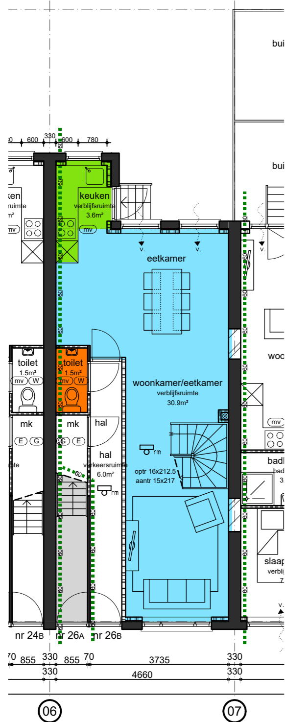
woning 26 B beganegrond nieuw
