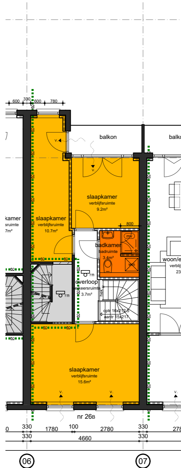
woning 26 B 1e verdieping nieuw
